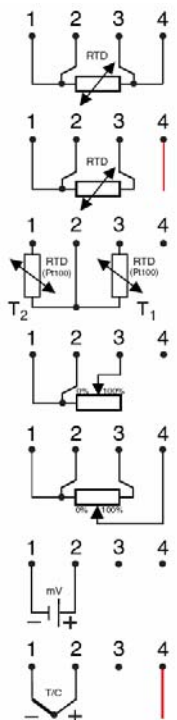
RTD 4-vodičové zapojení
